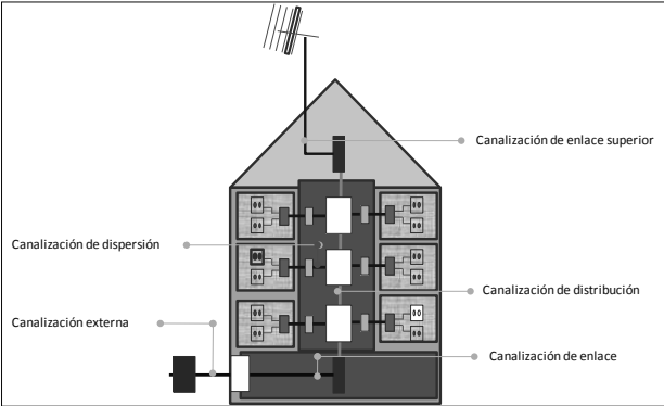
Gráfico 5. Estructura de la red de canalización
