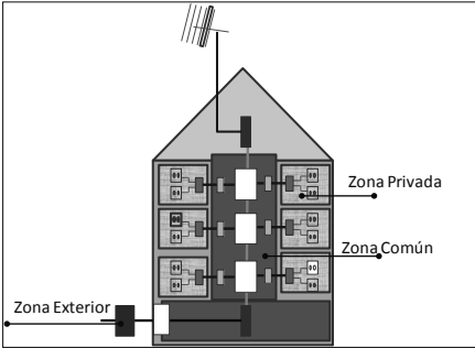
Gráfico 4. División por zonas de infraestructura
