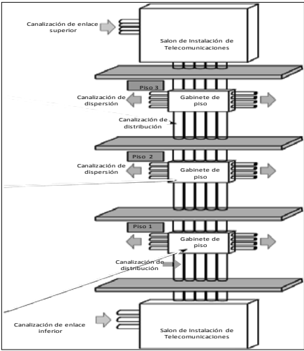
Gráfico 6. Esquema de canalización de distribución
